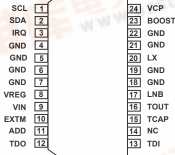
A8287SIB SOIC
