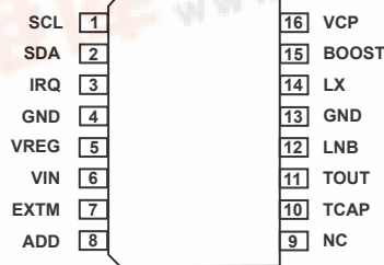
A8285SIB SOIC
