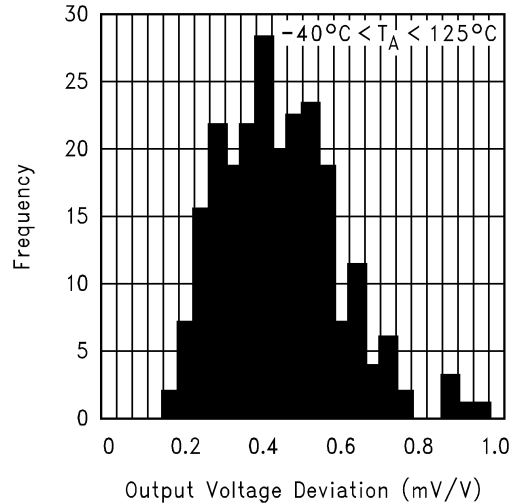
Thermal Hysteresis
