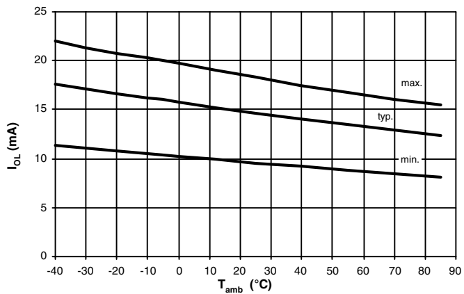
Figure 109. Output Low Current versus T amb , V DD = 6.5 V, V OL = 0.2 × V DD
