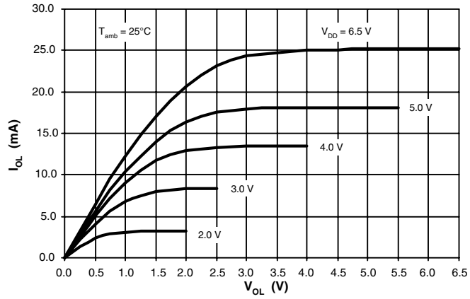
Figure 108. Output High Current versus T amb , V DD = 6.5 V, V OH = 0.8 × V DD
