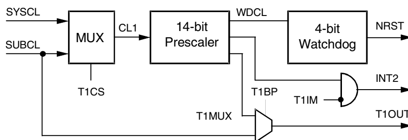
Figure 28. Timer 1 Module
