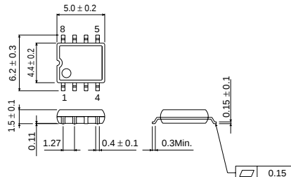
SOP8
