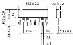
SIP8
