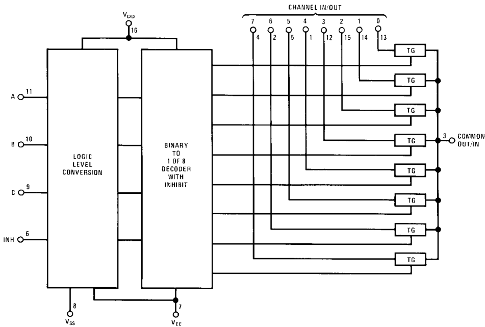
CD4051BC
