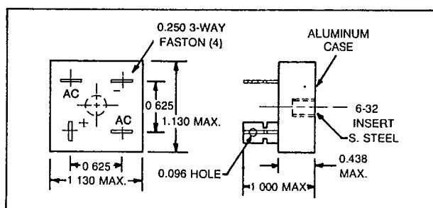
Case Style 3E
