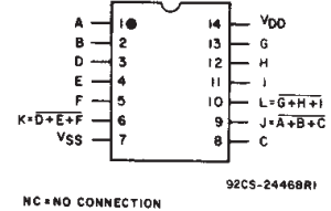
CD4025B
