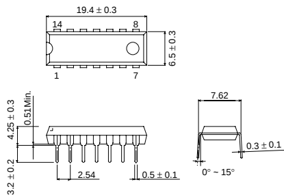
DIP14
