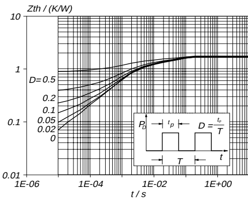
Fig.12. Transient thermal impedance. Z_{th\ j-mb} = f(t) ; parameter D = t_p/T
