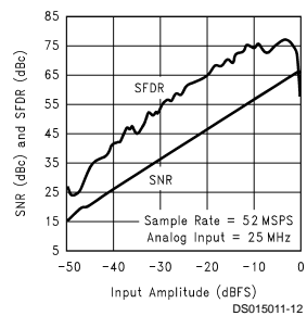
SNR and SFDR vs Input Amplitude
