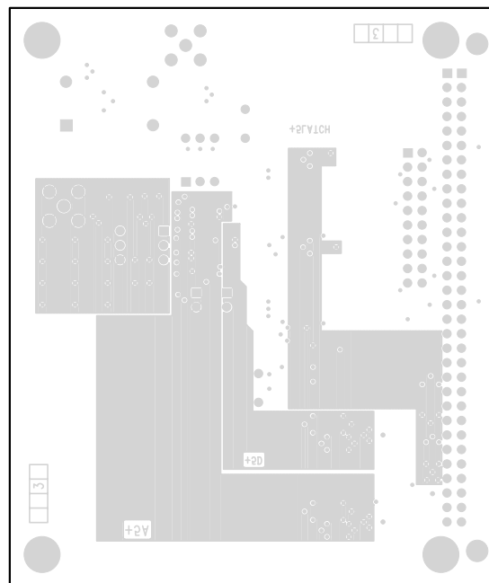
CLC5957PCASM Layer 3
