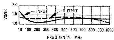
VSWR
