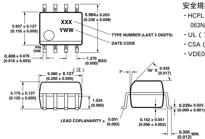
図3 . 8ピンミニフラットタイプ( HCPL-061A/061N/063A/063N )
