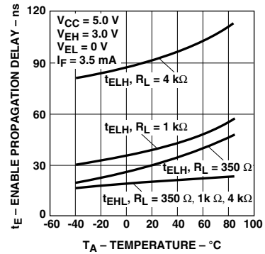
図16．インーブル伝達遅延—温度特性 ( HCPL-261A/-261N/-061A/-061N )
