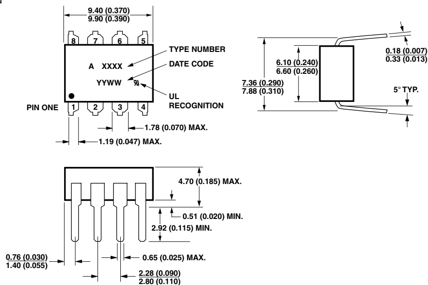
図1. 標準パッケージ寸法図 (HCPL-261A/261N/263A/263N)
