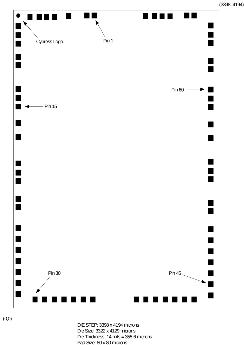
Figure 3-2. CY7C66113C DIE
