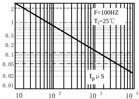
FIG-7 峰值脉冲电流与脉冲宽度关系曲线（最大值） Peak Pulse Current Versus Pulse duration (maximum values)
