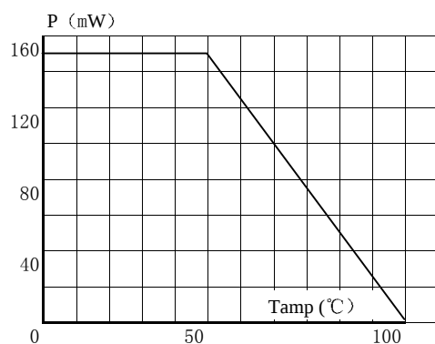
FIG -5 功耗环境温度关系曲线 (最大值) Power dissipation versus ambiept temperature( maximum values)
