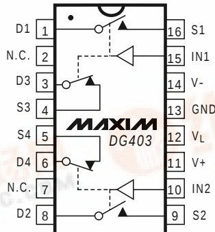
DIP/SO
