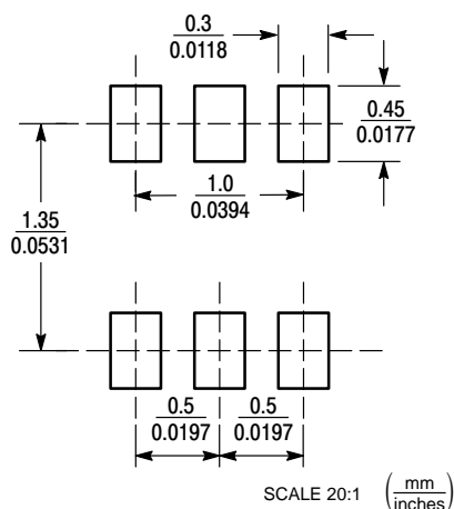
SOT-563
