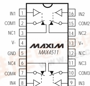
DIP/SO
