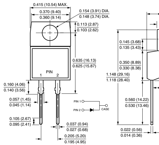
TO-220AC
