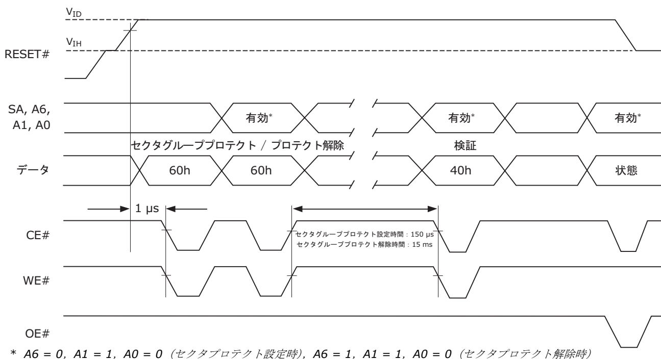
図 25. セクタ/セクタブロックプロテクトおよび プロテクト解除のタイミング図
