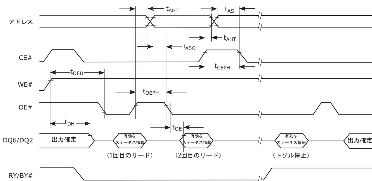
図 22. トグルビットのタイミング (自動アルゴリズム実行時)
