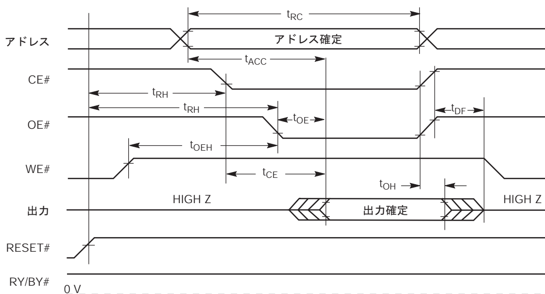
図 13. リード動作タイミング
