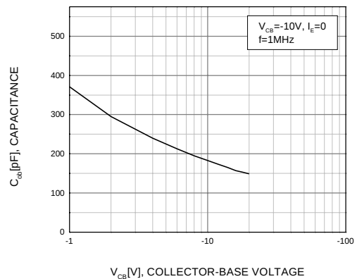
Fig. 6 Output Capacitance
