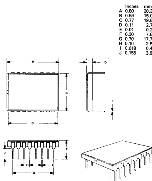
Fig. 6 FX003 D.I.L. Package
