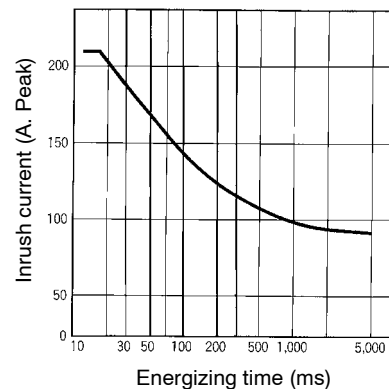
G3NE-220T(L)-US
