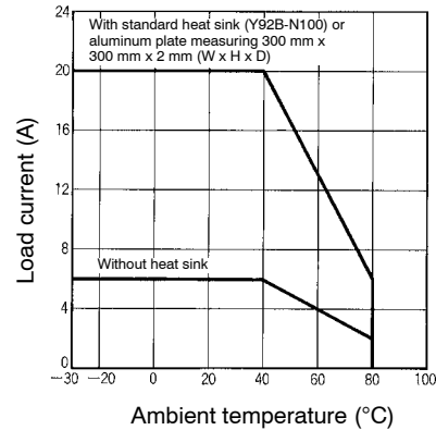
G3NE-220T(L)-US
