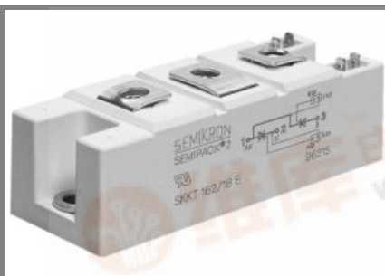
SEMIPACK ® 2
