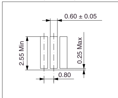
Detail A (Datum -A-)
