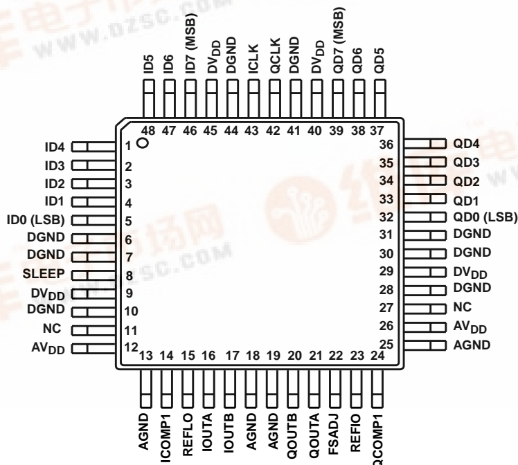
HI5628 (LQFP)
