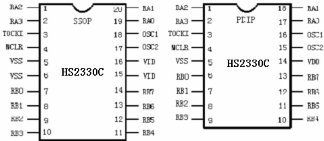
HS2330C 引脚说明表
