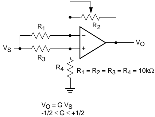
Attenuator
