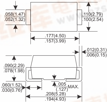
DO-214AC(SMA)
