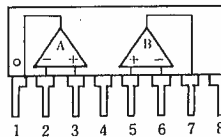
NJM4560L
