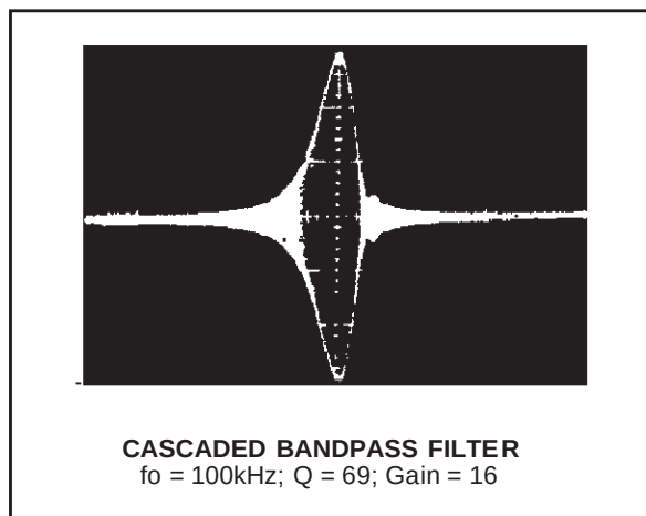
OUTPUT B
