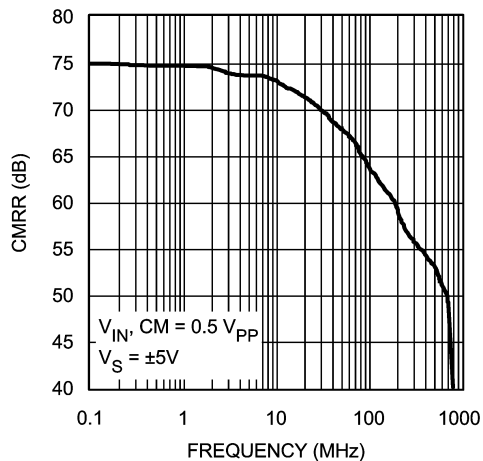
CMRR
