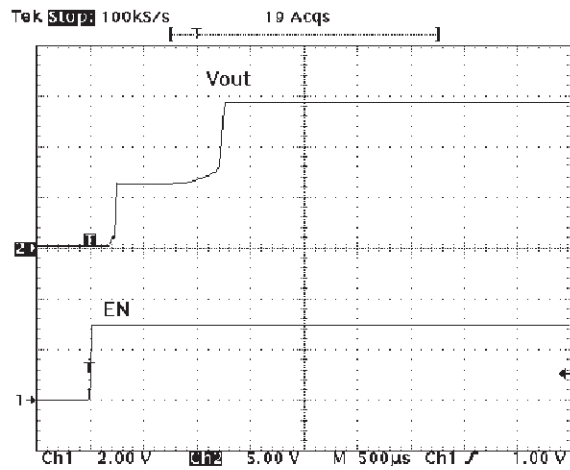
Enable Time
