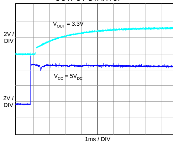
OUTPUT STARTUP
