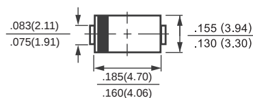
SMB (DO-214AA)
