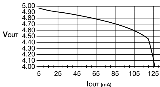
I_{OUT} - V_{OUT}
