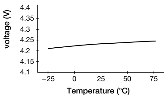
\overline{CS} detection voltage-Temperature
