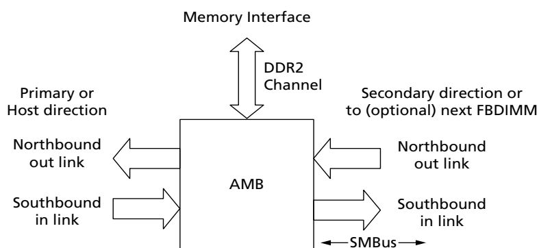
Figure 3: AMB Interface Block Diagram
