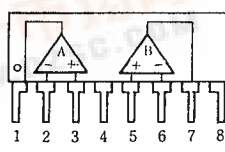
NJM2043L
