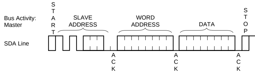
Byte Write (Figure 5).
