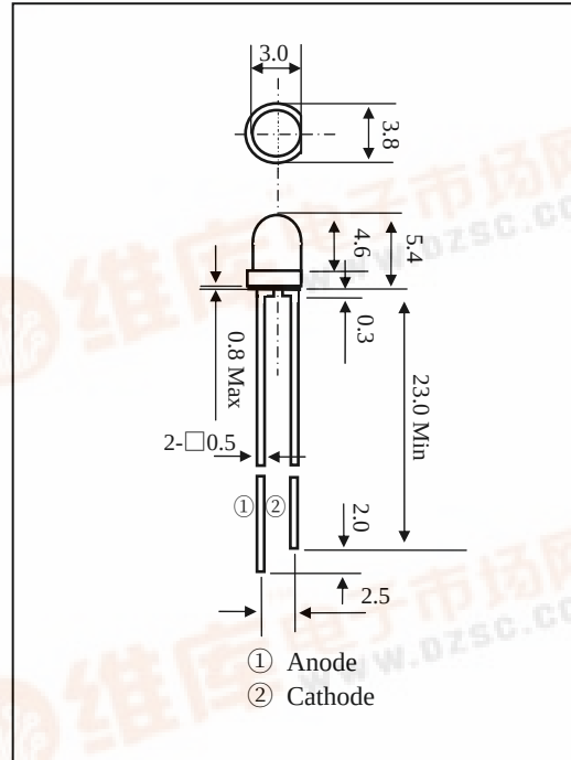
DIMENSIONS (Unit:mm)
