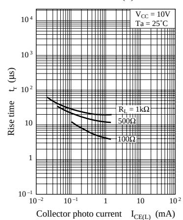
t_r - I_{CE(L)}
