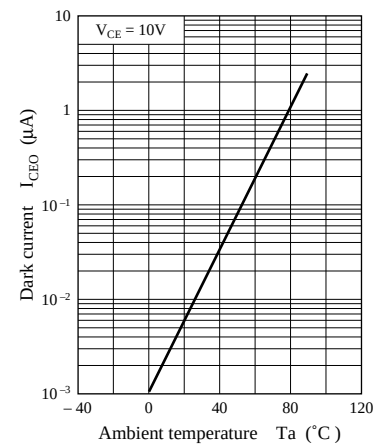
I_{CEO} - T_a
