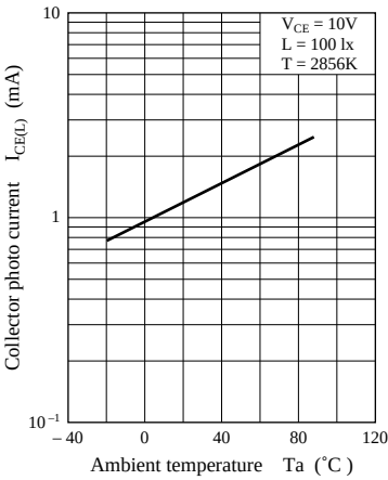
I_{CE(L)} - T_a
