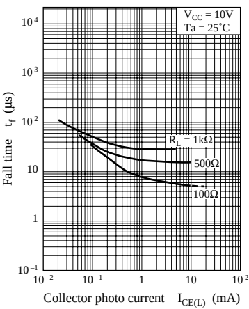
t_f - I_{CE(L)}
