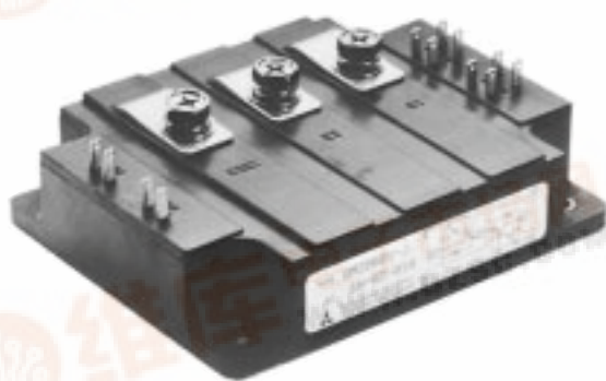
QM200DY-2H
