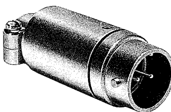
RM12BJB-2PH
