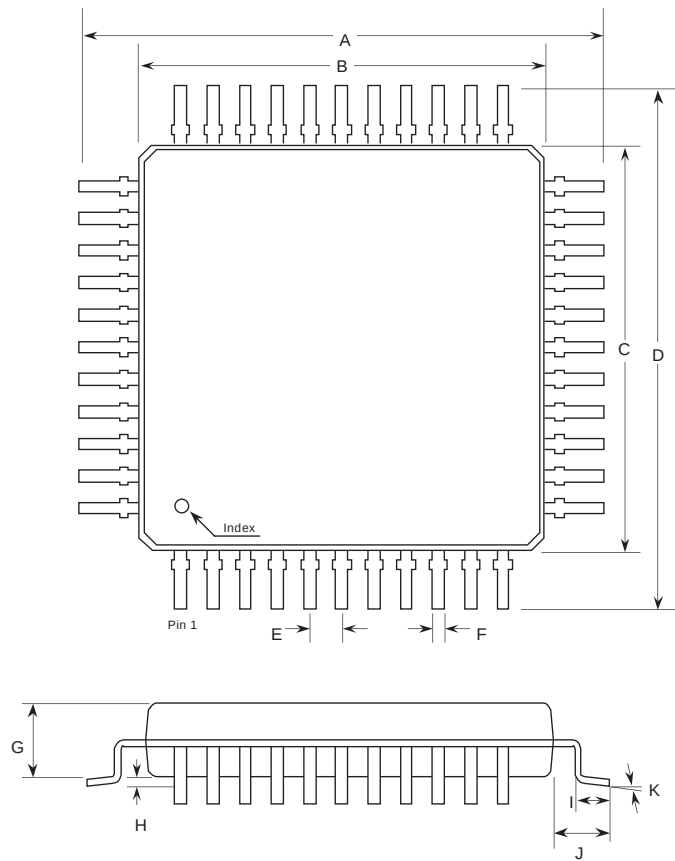
44L TQFP
