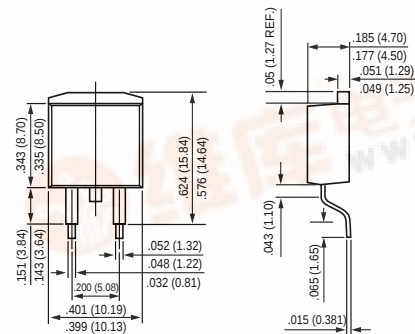
D2PAK
