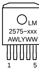
D 2 PAK D2T SUFFIX CASE 936A
