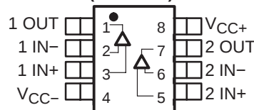
THS3122 SOIC (D) AND SOIC PowerPAD™ (DDA) PACKAGE (TOP VIEW)
