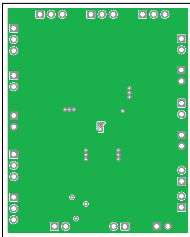
Figure 23. EVM Bottom Layer
