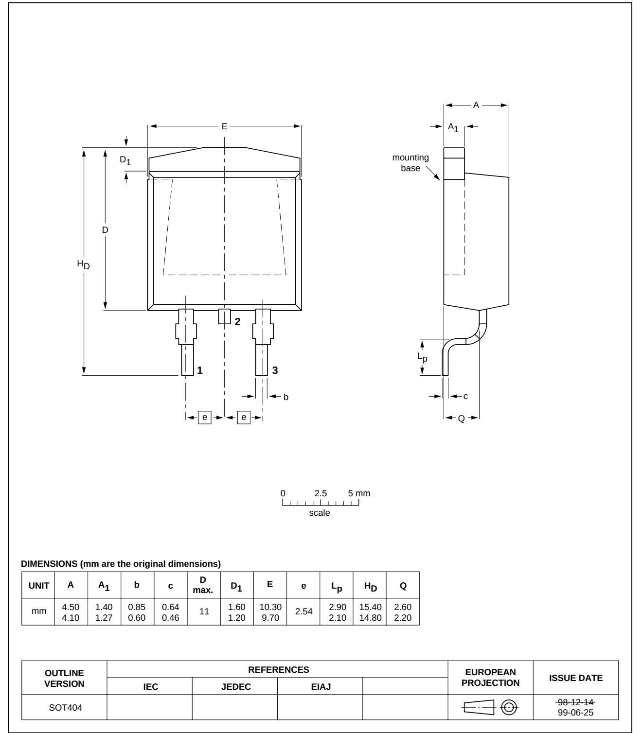
Fig 17. SOT404 (D 2 -PAK).
